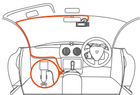
⑤ シガーソケットの取り付けと配線
